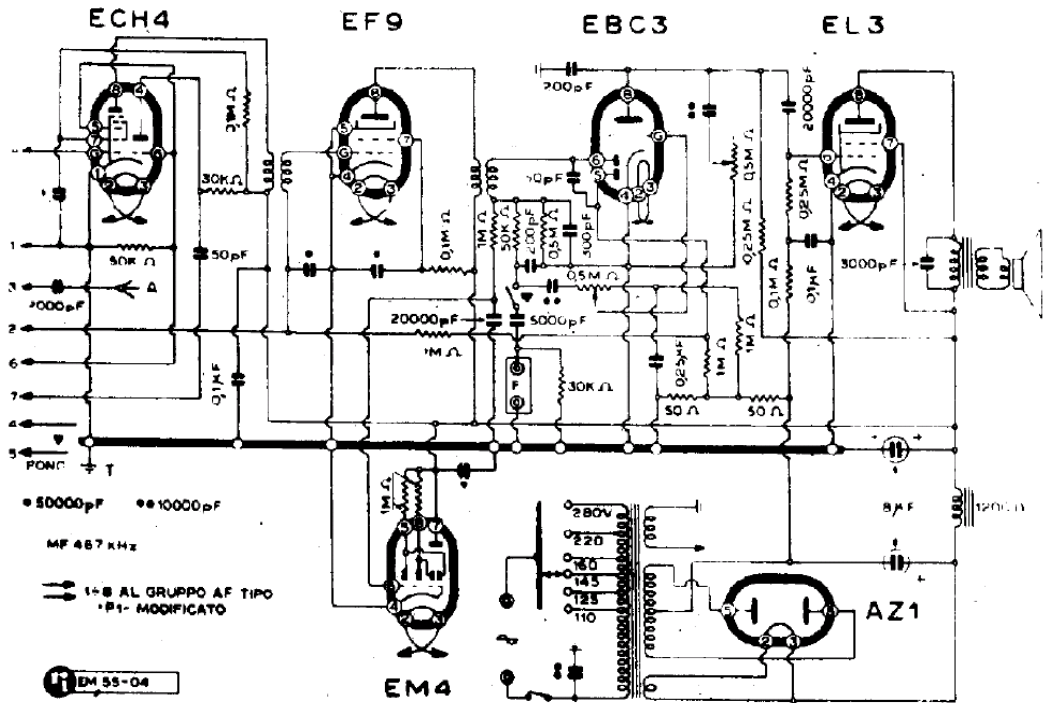
ELECTA RADIO - MOD. « ER 656 »
